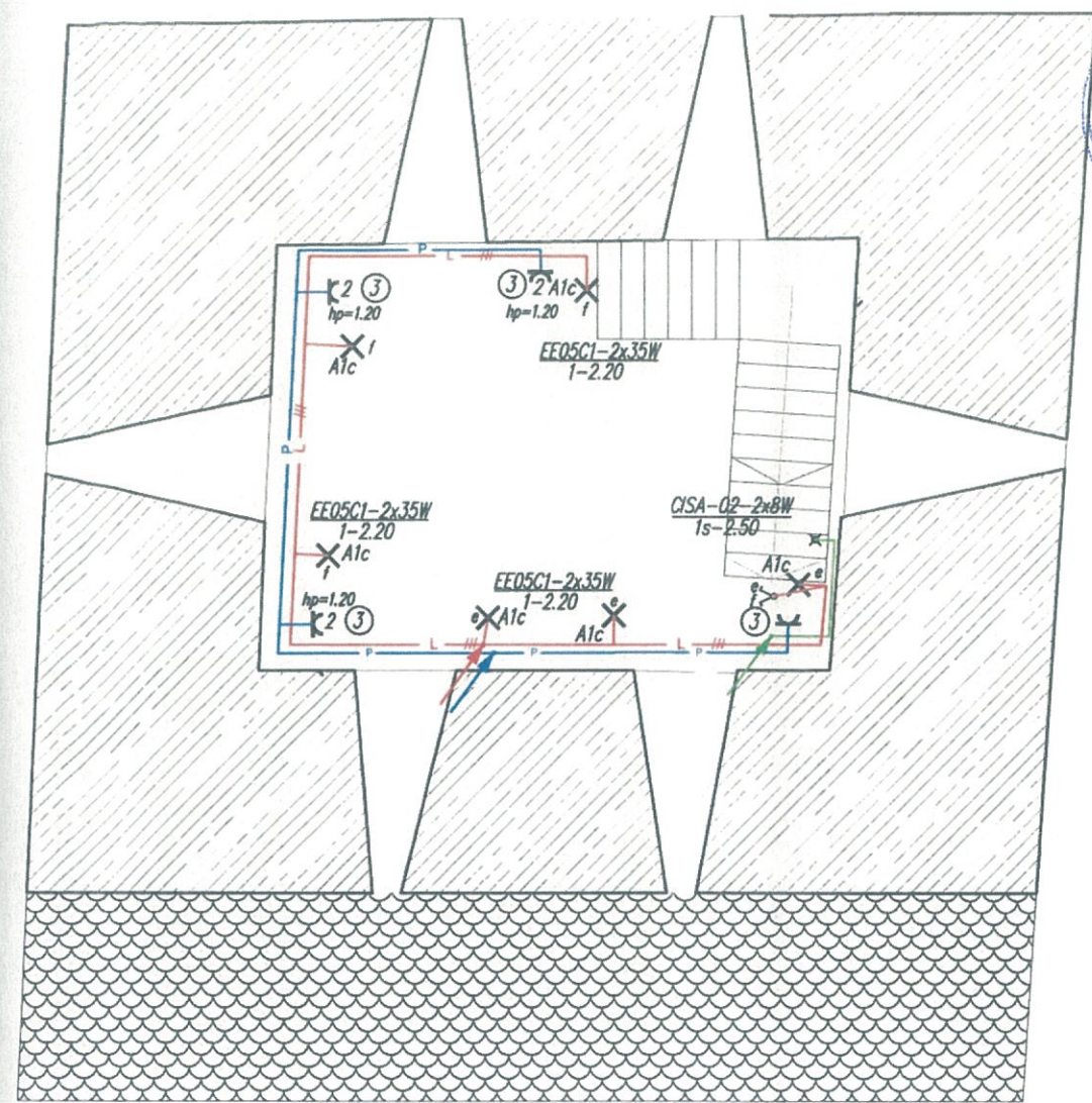
Plan cota +8.00
