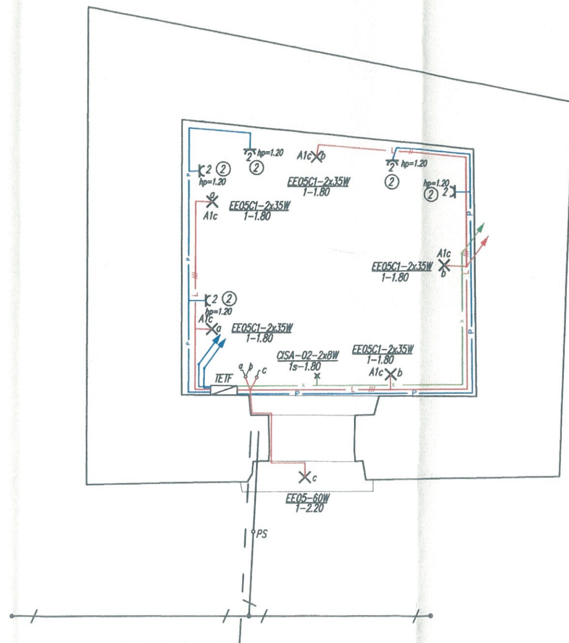
Plan cota +1.00m
