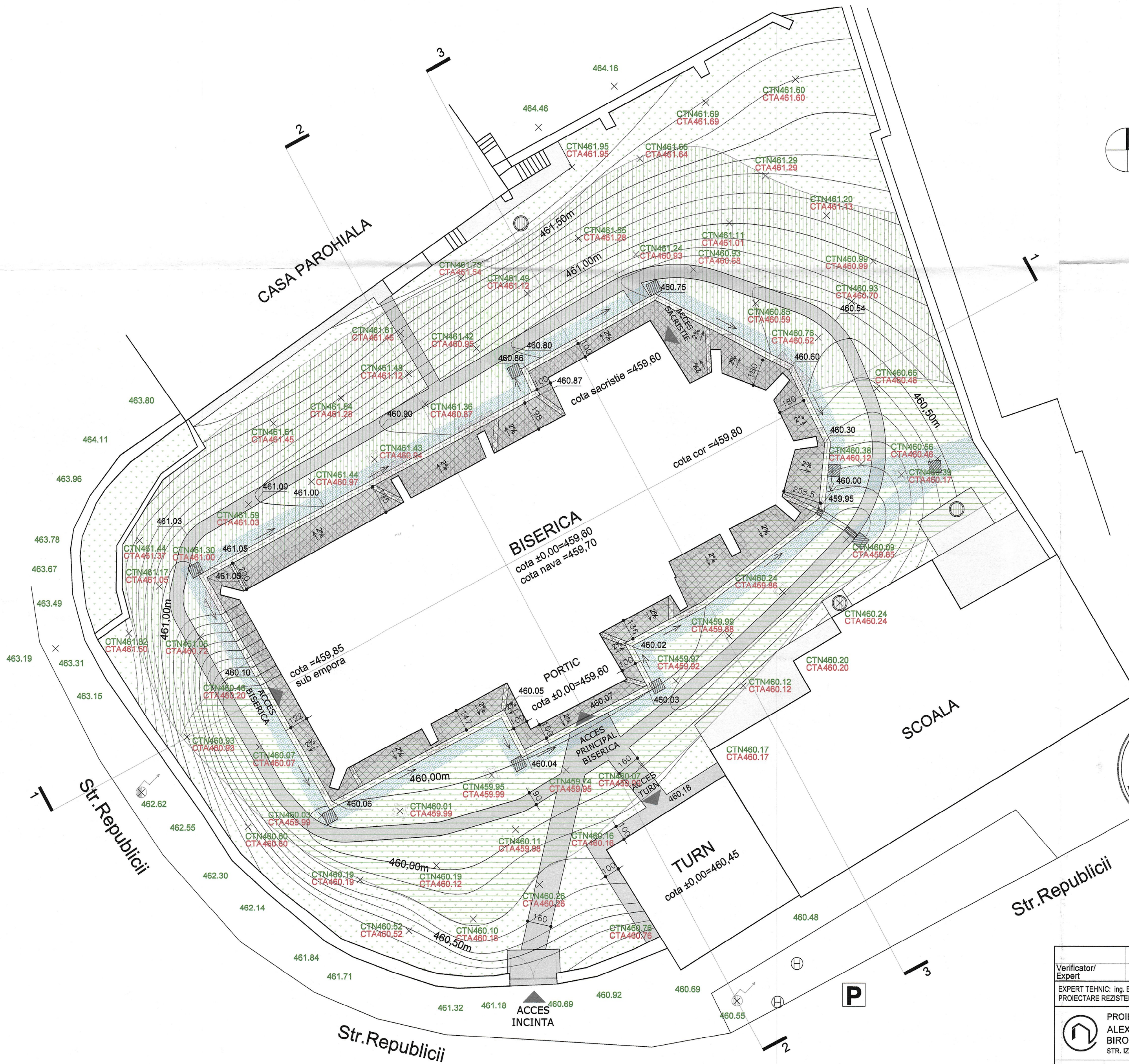
SISTEMATIZARE VERTICALA - PLAN INCINTA
