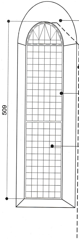
ELEVATIE SCARA 1/50
