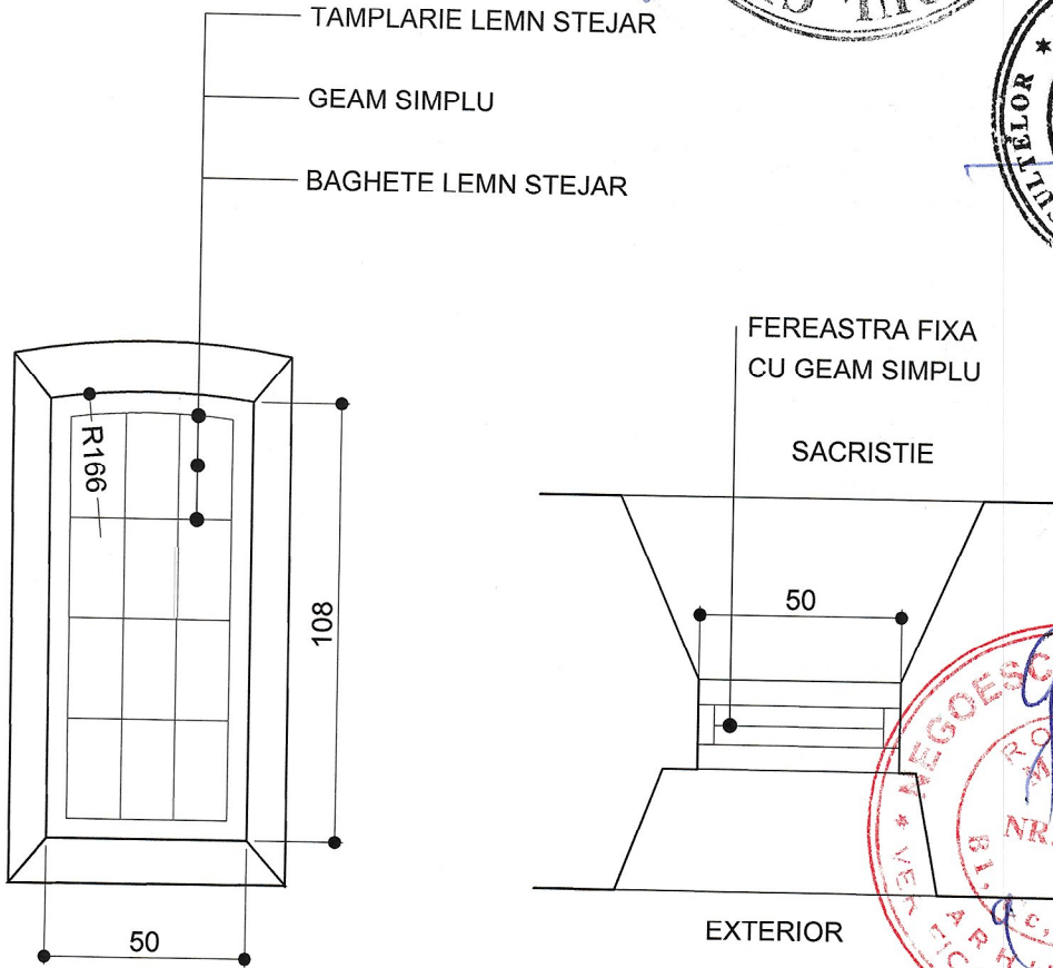
ELEVATIE SCARA 1/20
