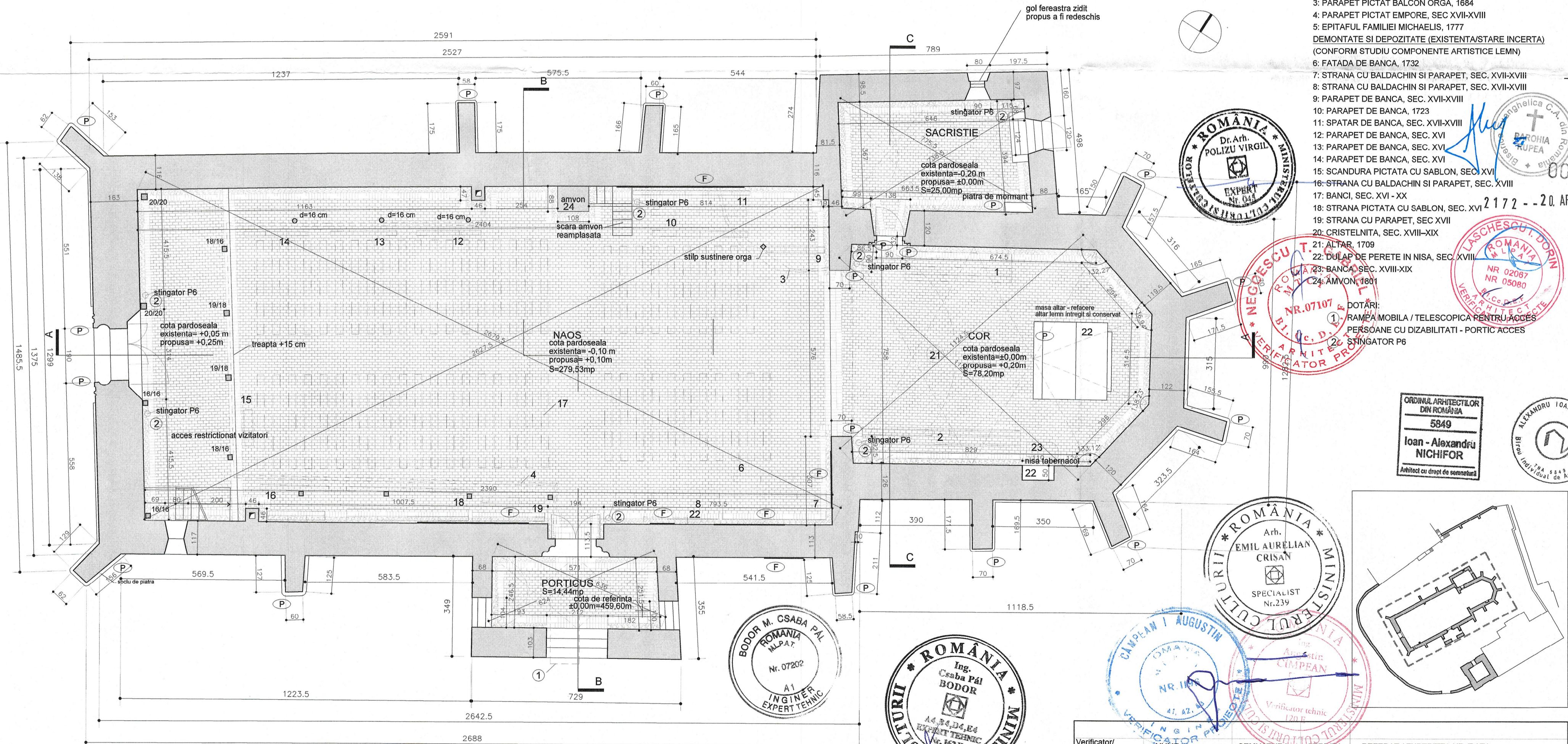
PLAN BISERICA COTA +1,20m
