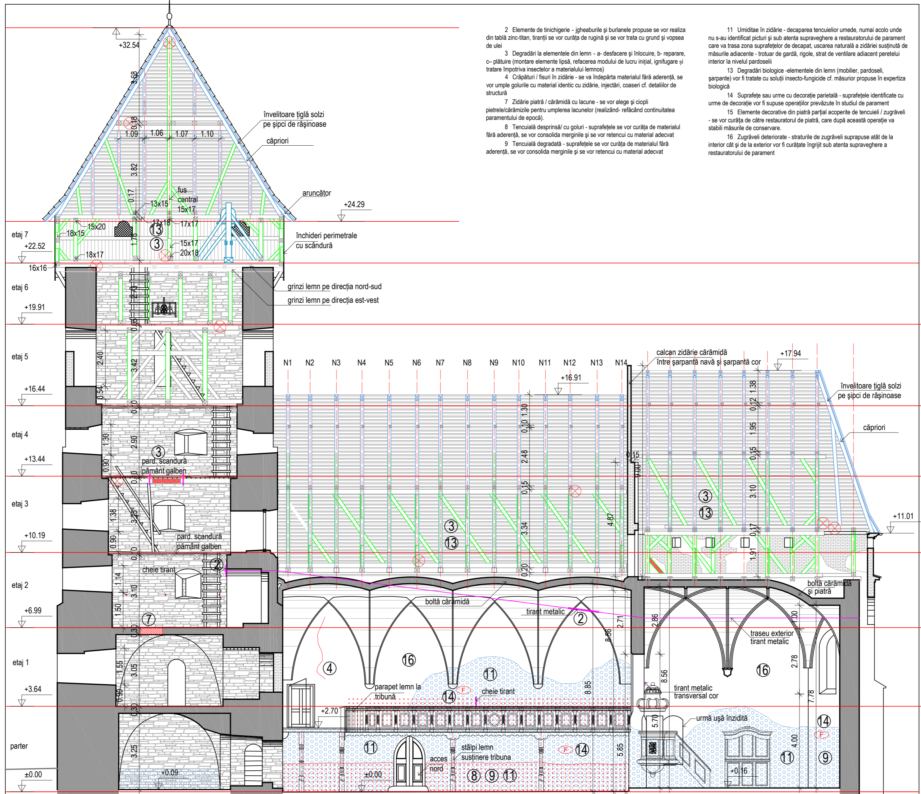
Secțiune longitudinală B-B vedere spre nord sc. 1/100
